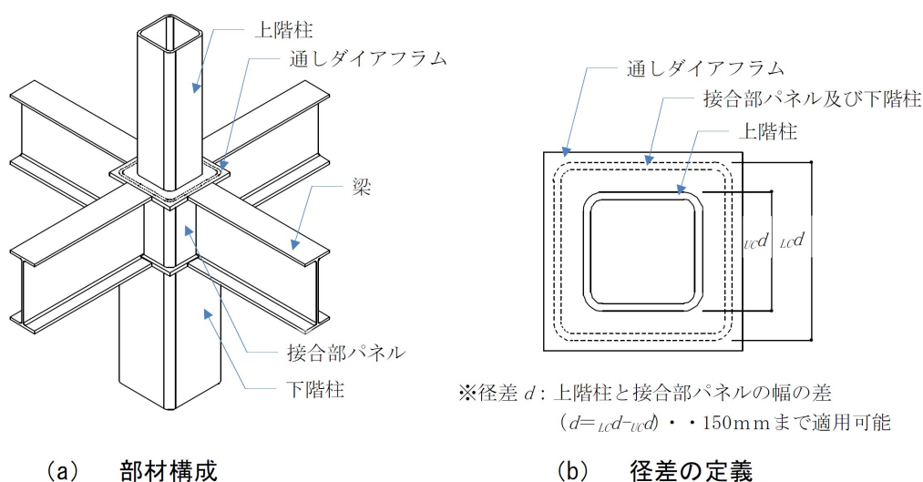
図-2 異幅柱接合部工法の概要
