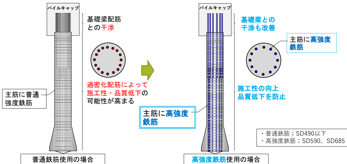
▲高強度鉄筋を主筋として用いた場合の効果
