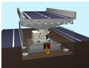
超低空頭場所打ち杭法工法
