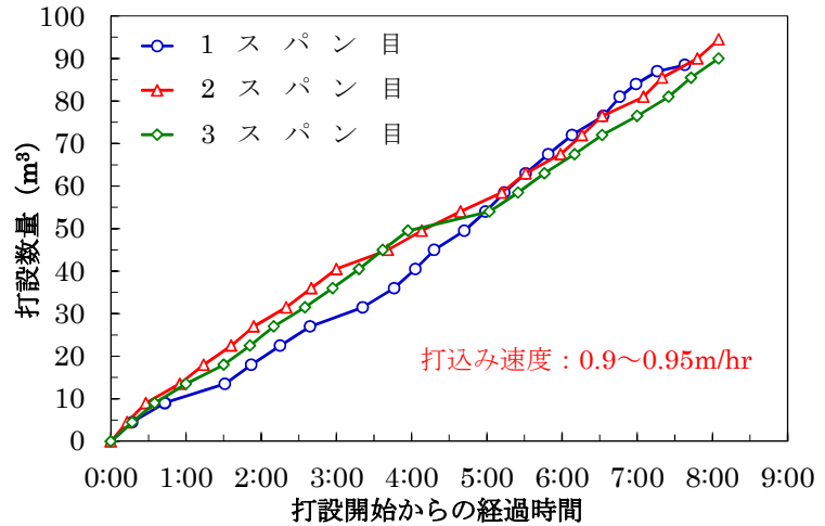
図-3 打設経過時間と打設数量の関係
