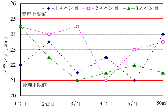
図-1 スランプ試験結果
